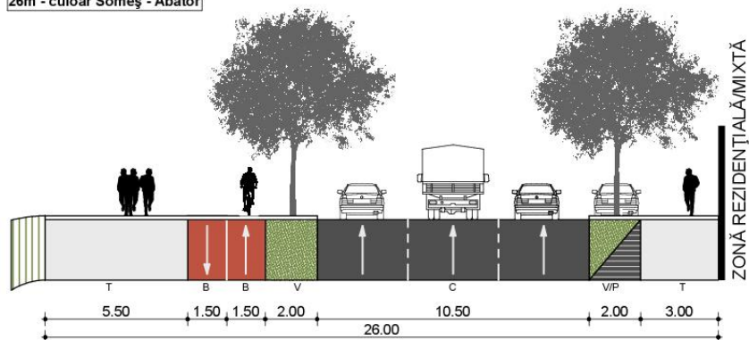
II.E 26m - culoar Someș - Abator
