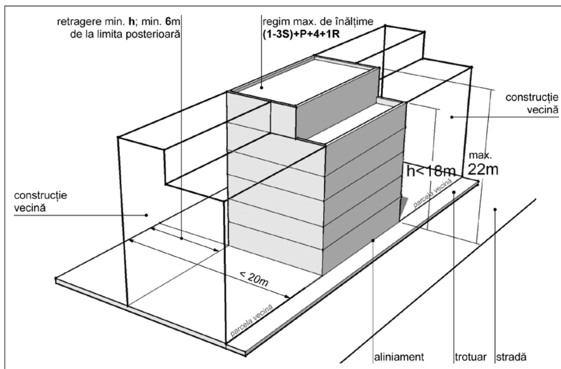
RrM1 - restructurare mixt locuire L < 20\text{ m}
