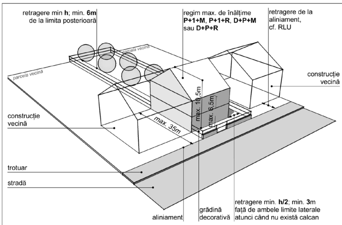
Lir - locuințe cu regim redus de înălțime cu caracter rural - cu calcan
