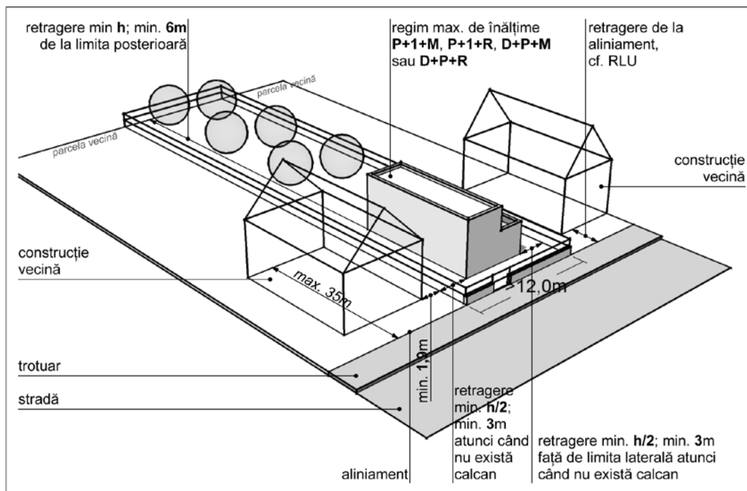
Lir - locuințe cu regim redus de înălțime cu caracter rural - front mai mare decât 12m - varianta 2 - fără calcan
