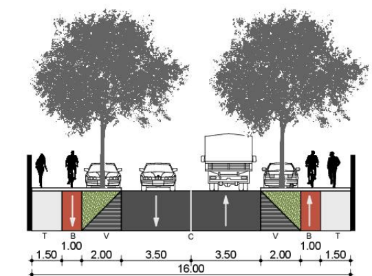
III.E 16 - rezidentiala - colectoare
