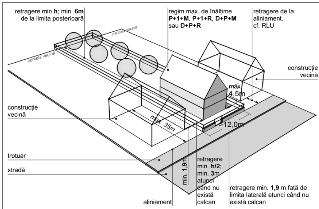
Lir - locuințe cu regim redus de înălțime cu caracter rural - front mai mare decât 12m - varianta 1 - fără calcan
