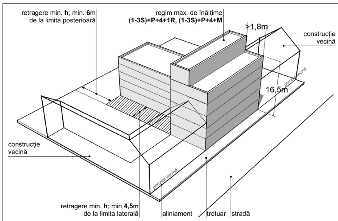
M1 - mixtă - cu un calcan
