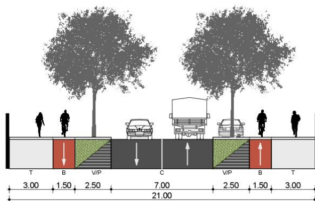
III.A 21m - zona mixta
