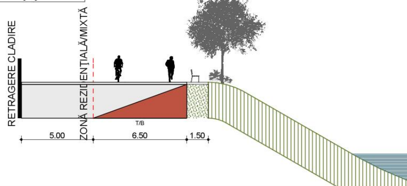
IV.3 8m - alee pietonală, mal stâng Someș între str. București și str. Traian
