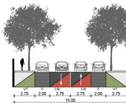
III.G 14m - zonă locuințe colective
