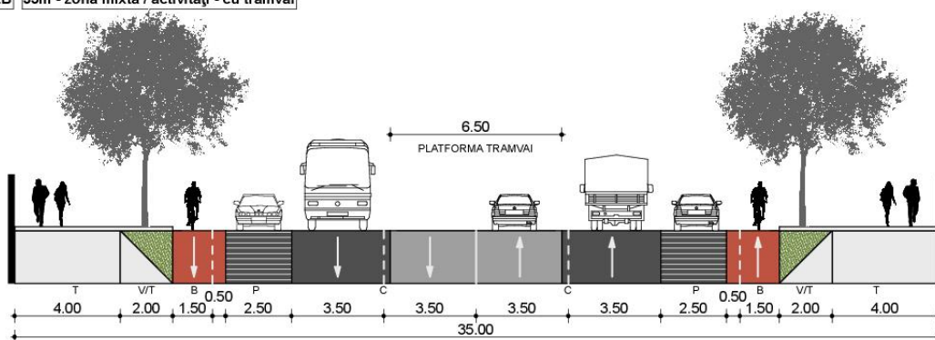
II.B 35m - zona mixtă / activități - cu tramvai
