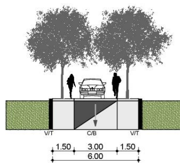
IV.2 6m - alee rezidențială / fundătură L&lt; 50m
