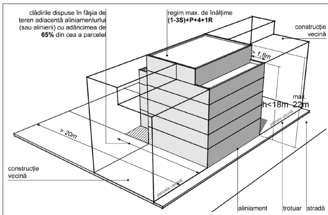
RrM1 - restructurare mixt locuire L > 20 m
