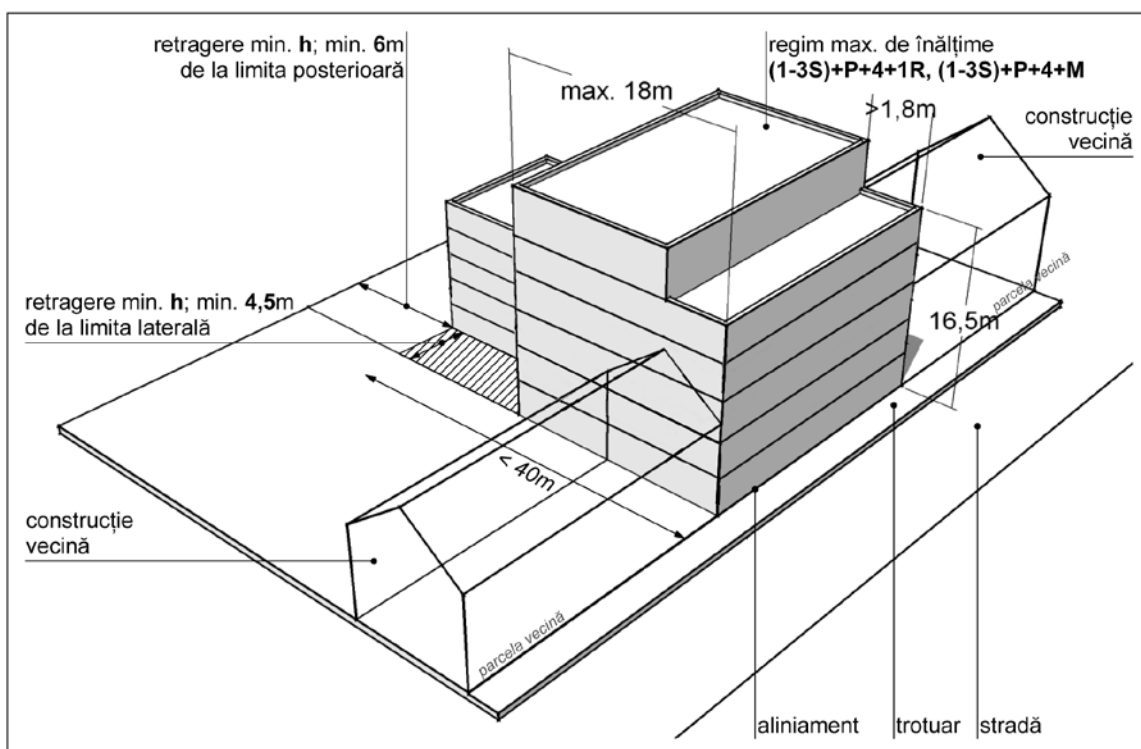
M1 - mixtă - cu două calcane
